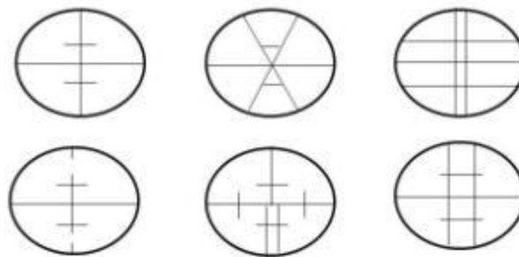
Fig: Stadia Diaphragm
