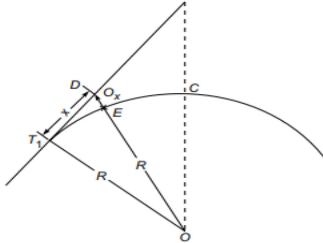
Fig: Radial Offset
